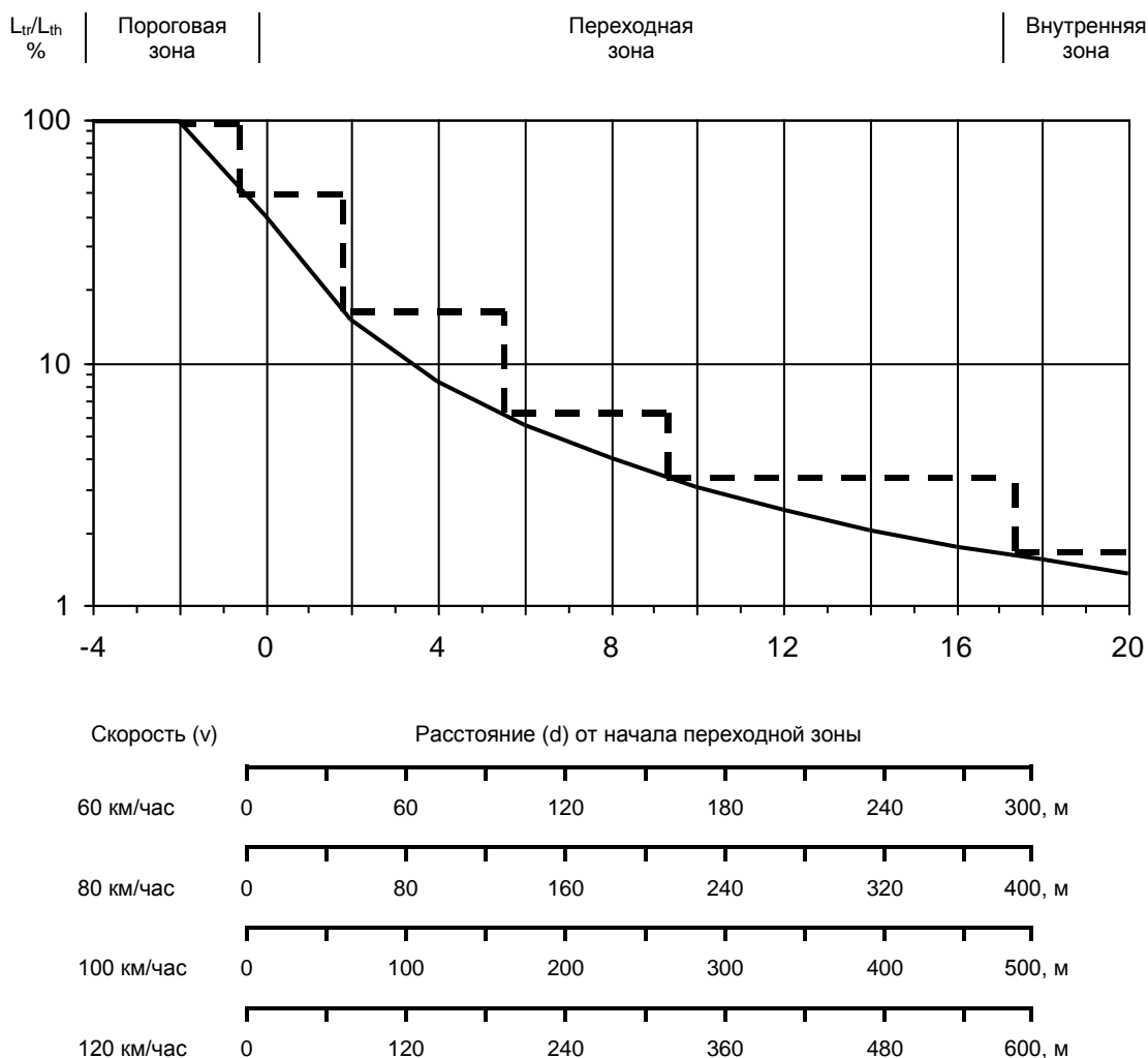
Рис.Ж.3. Кривая спада яркости дорожного покрытия в переходной зоне
