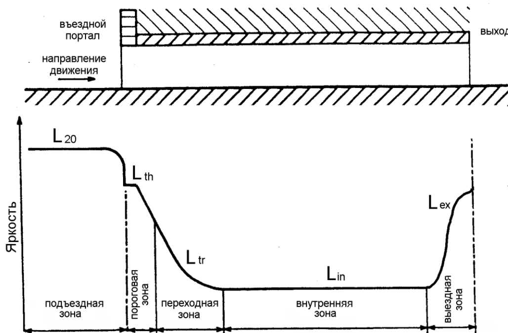
Рис.Ж.1 Яркостные зоны тоннеля в дневном режиме
