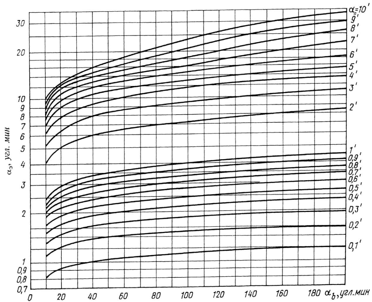
Рис. Г.2. Номограмма для определения эквивалентного размера протяженных объектов различения при расстояниях от глаза до объекта более 500 мм.
