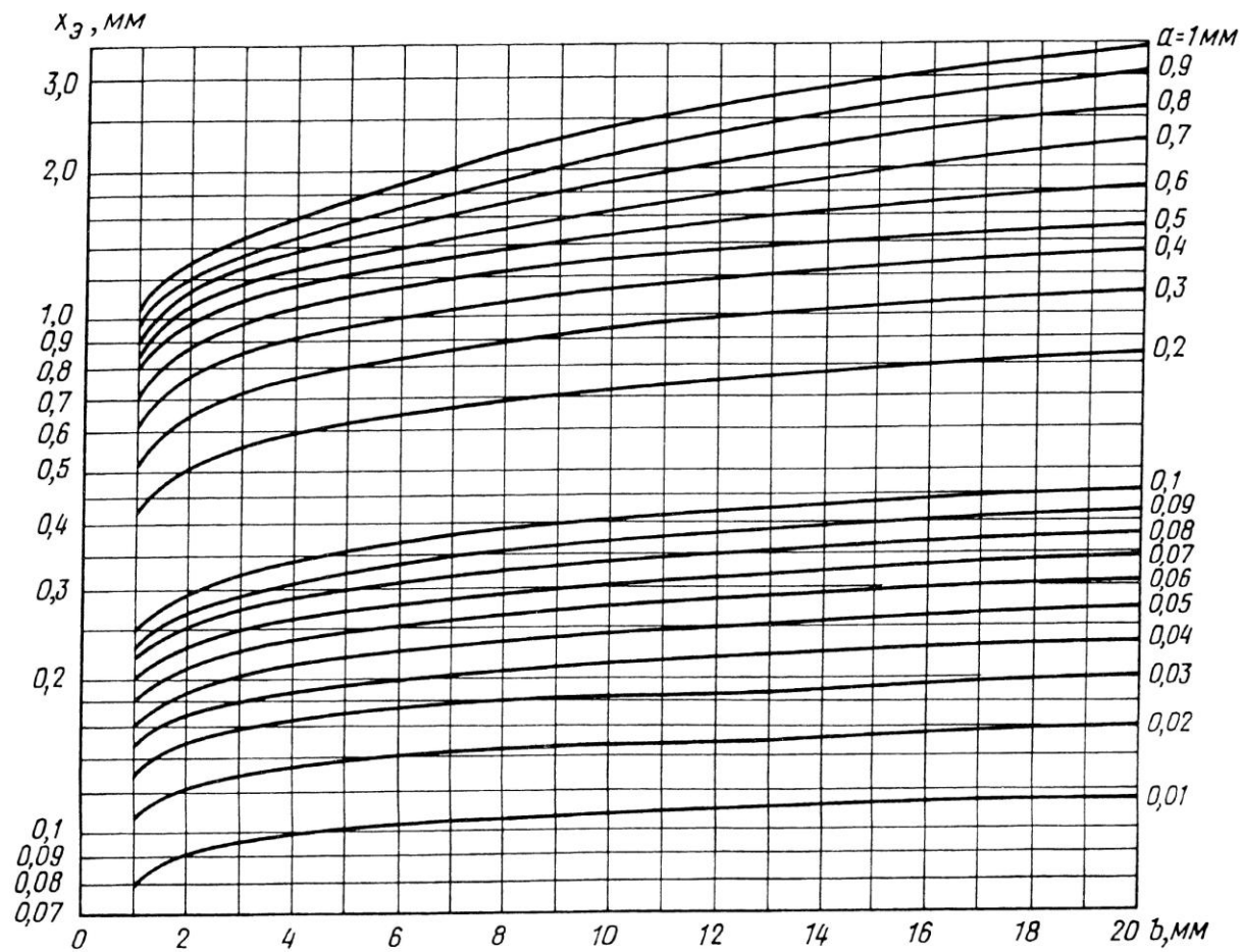
Рис. Г.1. Номограмма для определения эквивалентного размера протяженных объектов различения при расстояниях от глаза до объекта до 500 мм.
