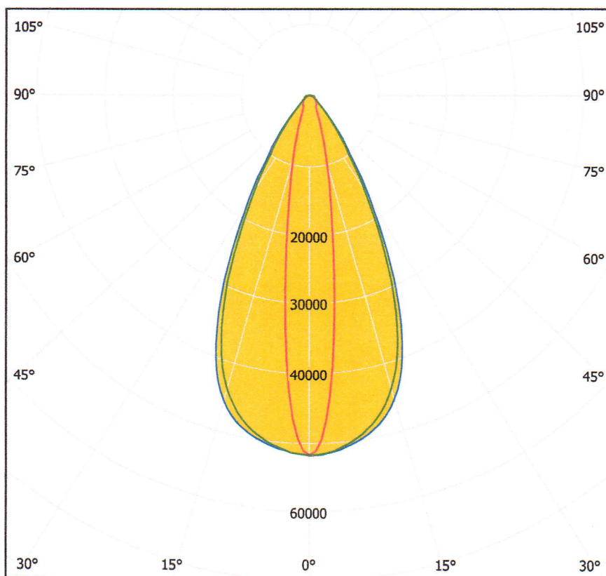
Рисунок 1 – КСС образца светильник светодиодный KEDR Stock LE-CBU-32-150-6599-67X в поперечной (C0-C180) (красная кривая), продольной (C90-C270) (синяя кривая) плоскостях и плоскости максимальной силы света (C98-C278) (зеленая кривая)
