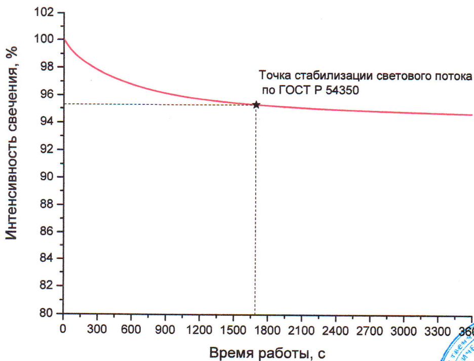
Рисунок 2 – График стабилизации светового потока образца светильник светодиодный KEDR Stock LE-CBU-32-150-6599-67X
